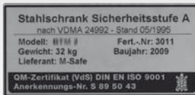
Musterplakette
